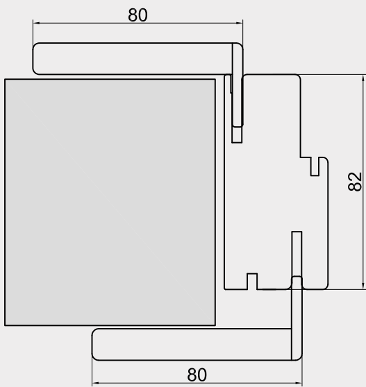
Per muro spesso da 8 a 9.5 cm For thickness from 8 to 9.5 cm Elargissement pour epaisseur de mur de 8 à 9.5 cm Expansión pared de 8 a 9.5 cm
