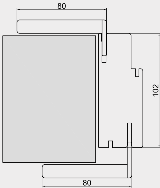
Per muro spesso da 10 a 11.5 cm For thickness from 10 to 11.5 cm Elargissement pour epaisseur de mur de 10 à 11.5 cm Expansión pared de 10 a 11.5 cm
