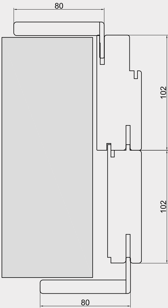
Allargamento per muro spesso da 20 a 21.5 cm
