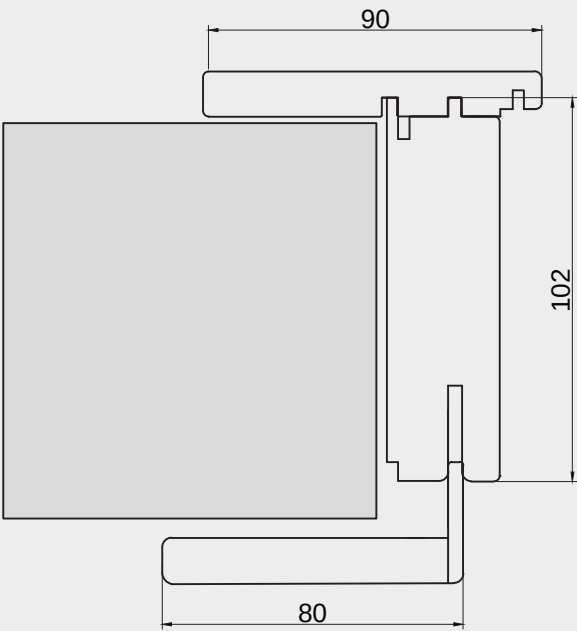
Per muro spesso da 9.5 a 11 cm For thickness from 9.5 to 11 cm Elargissement pour epaisseur de mur de 9.5 à 11cm Expansión pared de 9.5 a 11 cm
