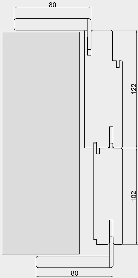
Allargamento per muro spesso da 22 a 23.5 cm
