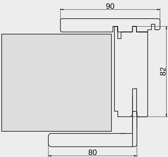
Per muro spesso da 7.5 a 9 cm For thickness from 7.5 to 9 cm Elargissement pour epaisseur de mur de 7.5 à 9 cm Expansión pared de 7.5 a 9 cm
