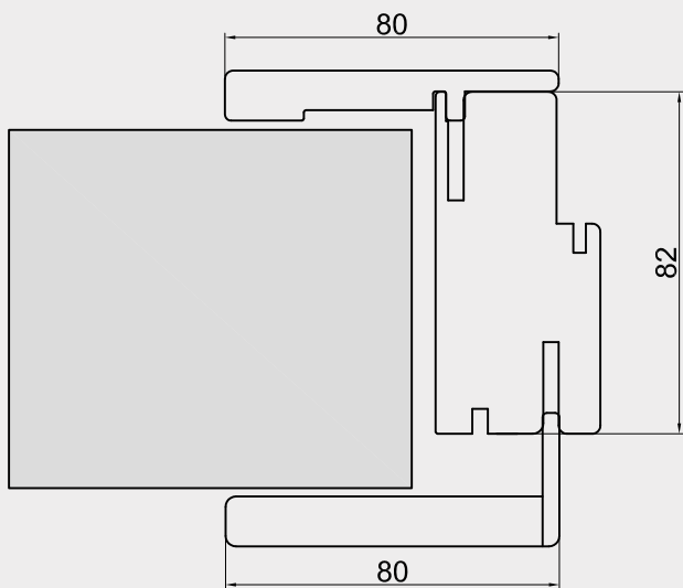
Per muro spesso da 7.5 a 9 cm For thickness from 7.5 to 9 cm Elargissement pour epaisseur de mur de 7.5 à 9 cm Expansión pared de 7.5 a 9 cm
