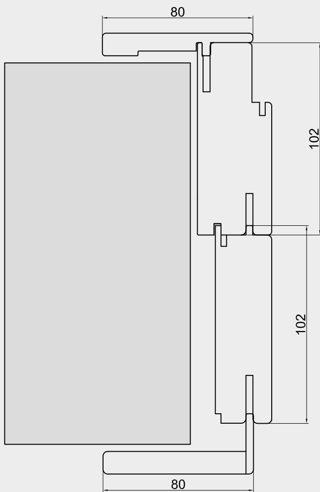
Allargamento per muro spesso da 19.5 a 21 cm Footing for thickness from 19.5 to 21 cm Elargissement pour épaisseur de mur de 19.5 à 21 cm Expansión pared de 19.5 a 21 cm
