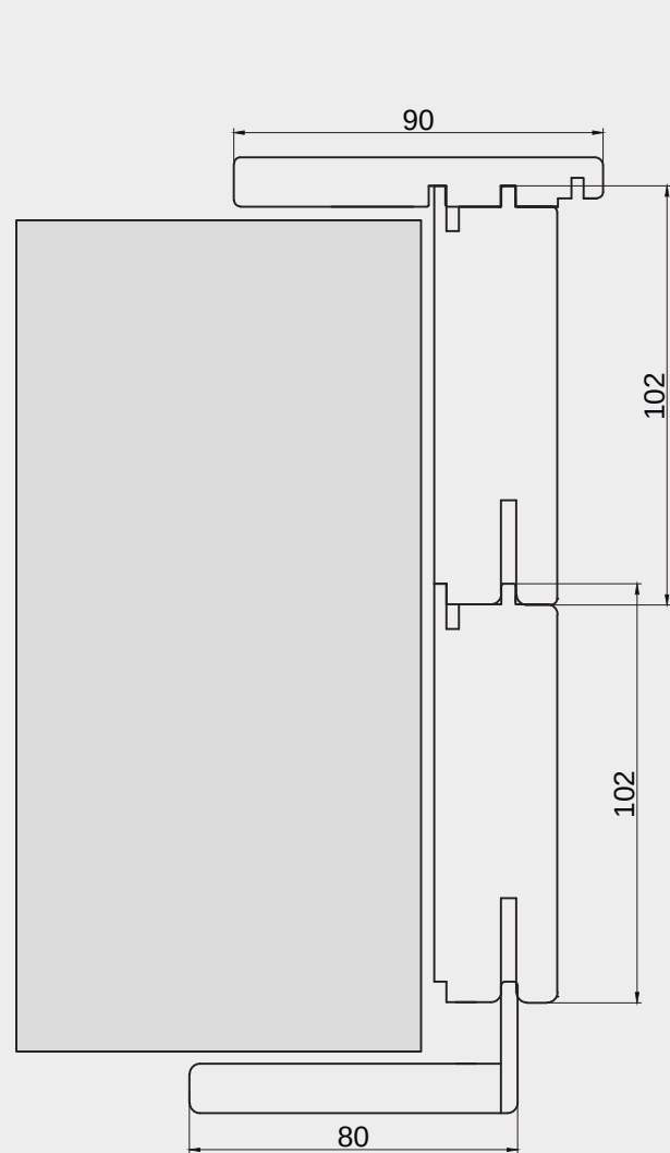
Allargamento per muro spesso da 19.5 a 21 cm Footing for thickness from 19.5 to 21 cm Elargissement pour epaisseur de mur de 19.5 à 21 cm Expansión pared de 19.5 a 21 cm
