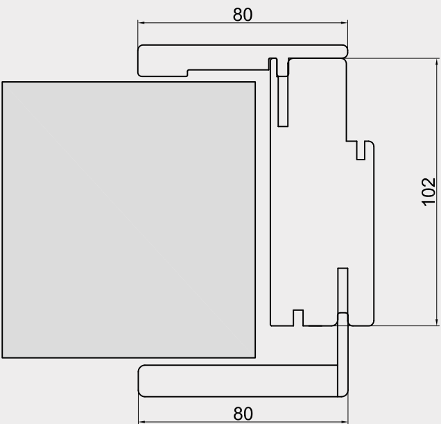
Per muro spesso da 9.5 a 11 cm For thickness from 9.5 to 11 cm Elargissement pour epaisseur de mur de 9.5 à 11 cm Expansión pared de 9.5 a 11 cm
