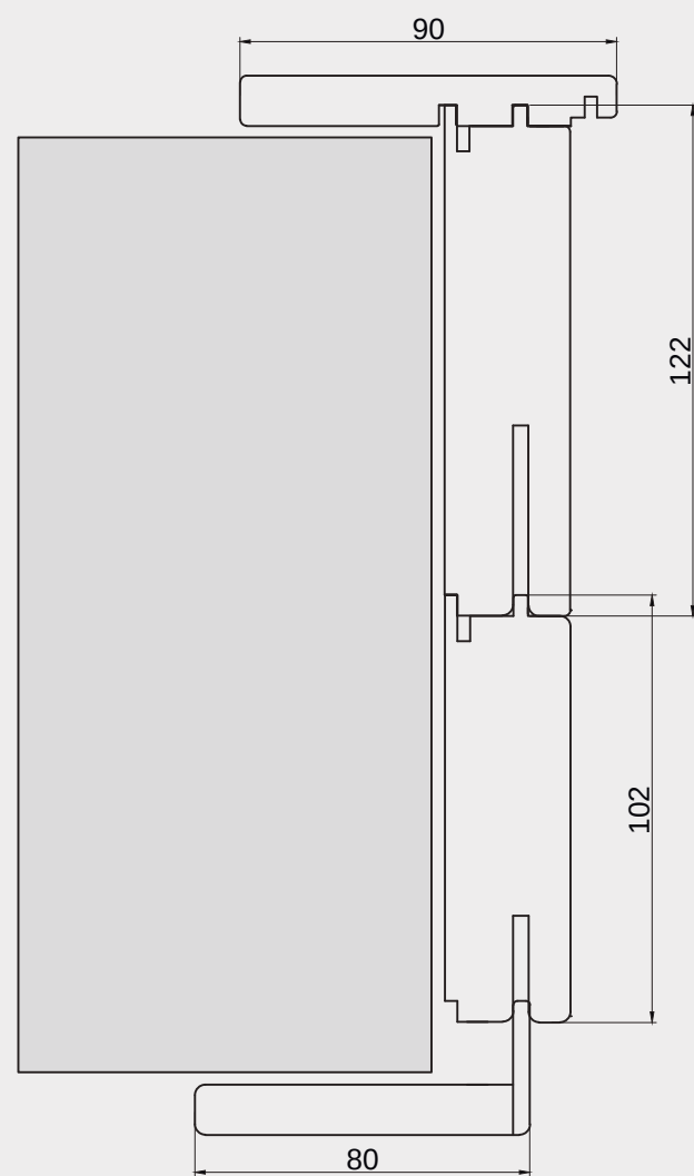
Allargamento per muro spesso da 21.5 a 23 cm Footing for thickness from 21.5 to 23 cm Elargissement pour epaisseur de mur de 21.5 à 23 cm Expansión pared de 21.5 a 23 cm
